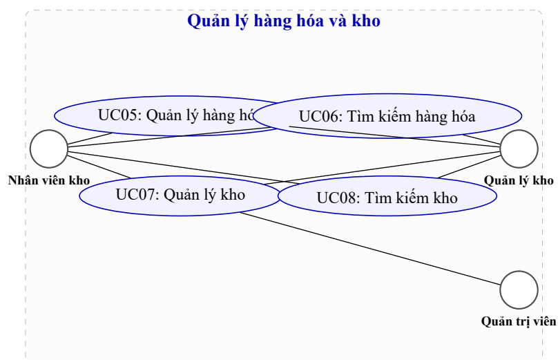
Hình 3.7: Sơ đồ use case phân rã – Quản lý hàng hóa và kho
