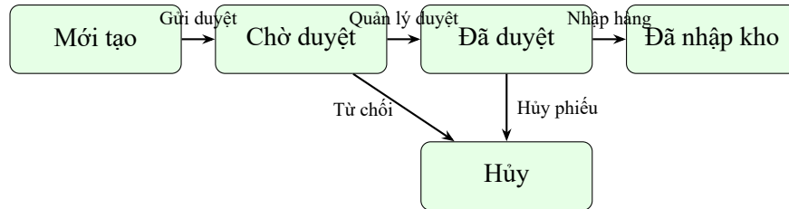
Hình 5.5: State Machine Diagram – Trạng thái phiếu nhập kho
