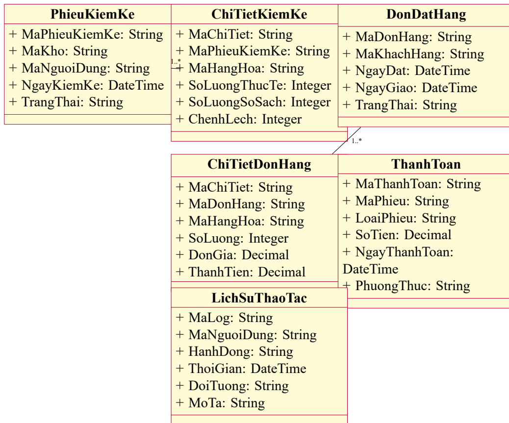
Hình 4.3: Sơ đồ lớp kiểm kê, đơn hàng và thanh toán
