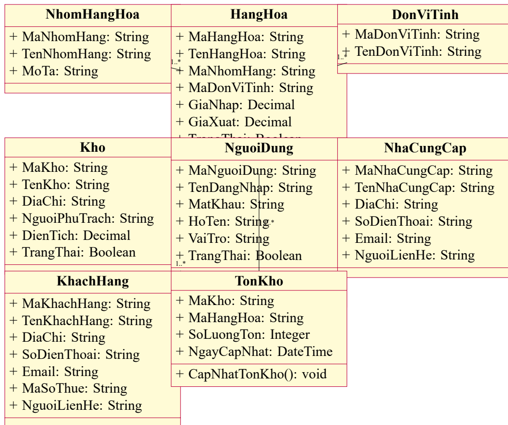
Hình 4.1: Sơ đồ lớp danh mục (Master Data)
