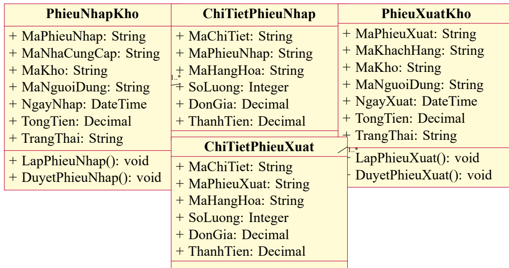
Hình 4.2: Sơ đồ lớp nghiệp vụ nhập xuất kho
