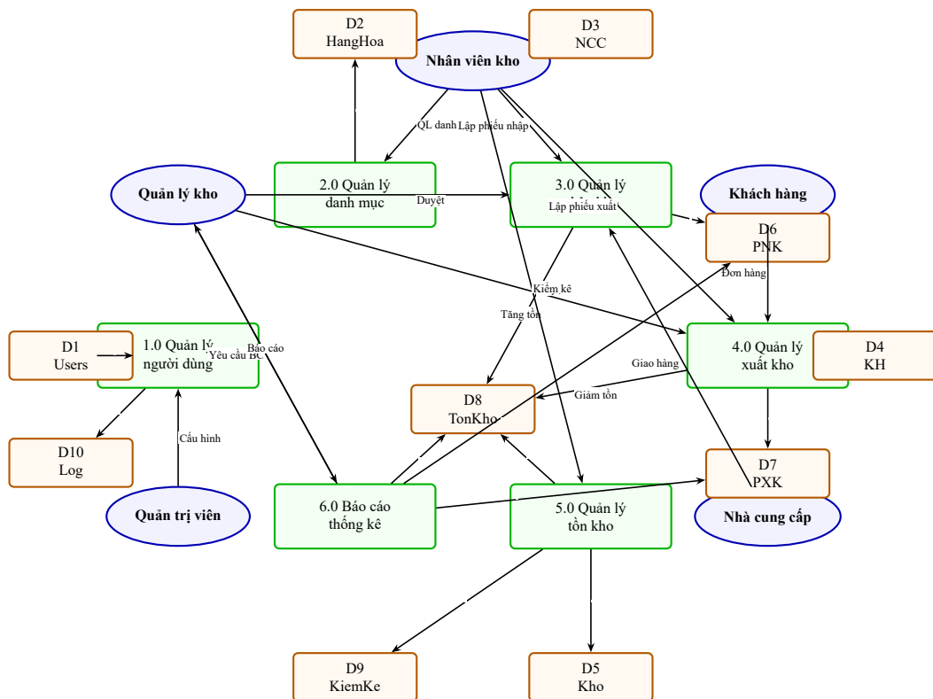
Hình 3.3: DFD cấp 1 – Phân rã các luồng dữ liệu trong hệ thống quản lý kho hàng
