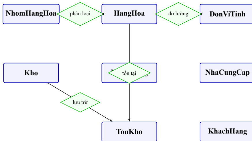
Hình 7.1: Sơ đồ ERD – Danh mục (Master Data)
